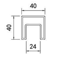
FSG04 不锈钢 SS T=1.5mm
