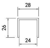
FSG07 不锈钢 SS T=2mm
