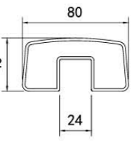
FSG03 铝 Alu T=2mm
