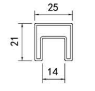
FSG08 不锈钢 SS T=1.2mm
