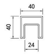
FSG01 铝 Alu T=2mm
